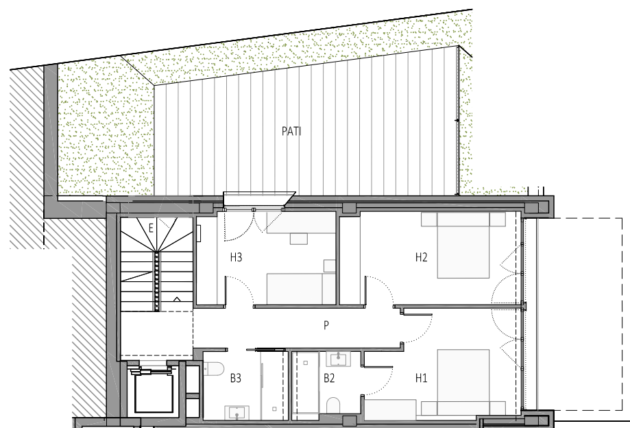
PLANTA PRIMERA
