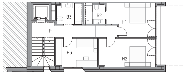
PLANTA PRIMERA
