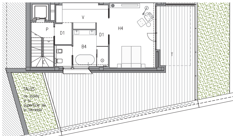
PLANTA BAIXA
